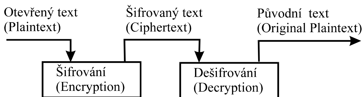
Figure 0.1 Šifrování (Encryption)
