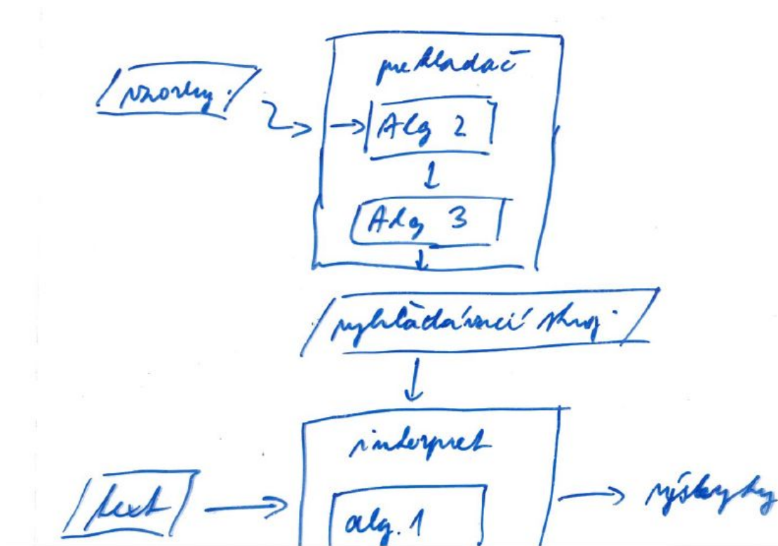
Obrázek 1: Celkové schéma algoritmu
