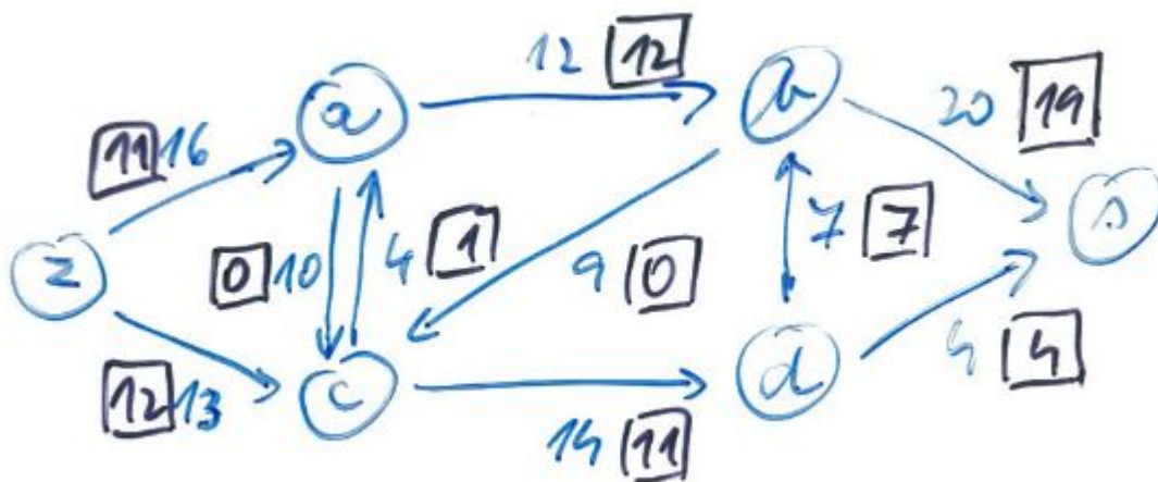
Obrázek 10: Síť: Modrou kapacitu, černou tok velikosti 23
